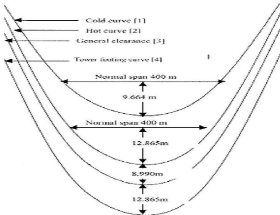
Fig 2.8- Sag Template
